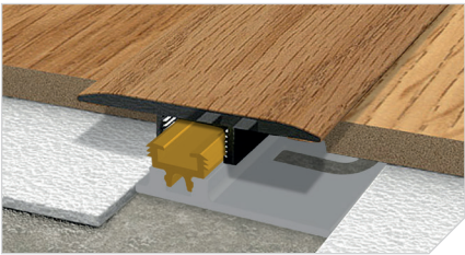
KIT GIUNTO DI DILATAZIONE + BASE PVC ANTIURTO per pavimenti con spess. da 5 a 7 mm rivestito con film digitale decoro coordinato
