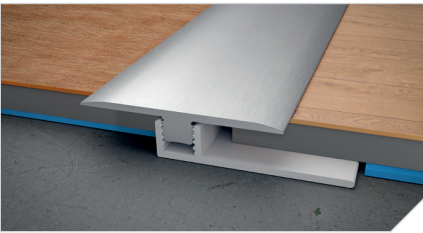
KIT GIUNTO DI DILATAZIONE + BASE PVC ANTIURTO per pavimenti con spess. da 5 a 7 mm in argento satinato
