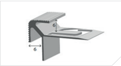
PARAGRADINO IN ALLUMINIO ANODIZZATO per pavimenti con spess. da 6 mm arrotondato e rigato
