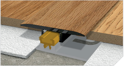
KIT GIUNTO DI DILATAZIONE + BASE ALLUMINIO ANTIURTO per pavimenti con spess. da 7 a 8 mm rivestito con film digitale deco coordinato
